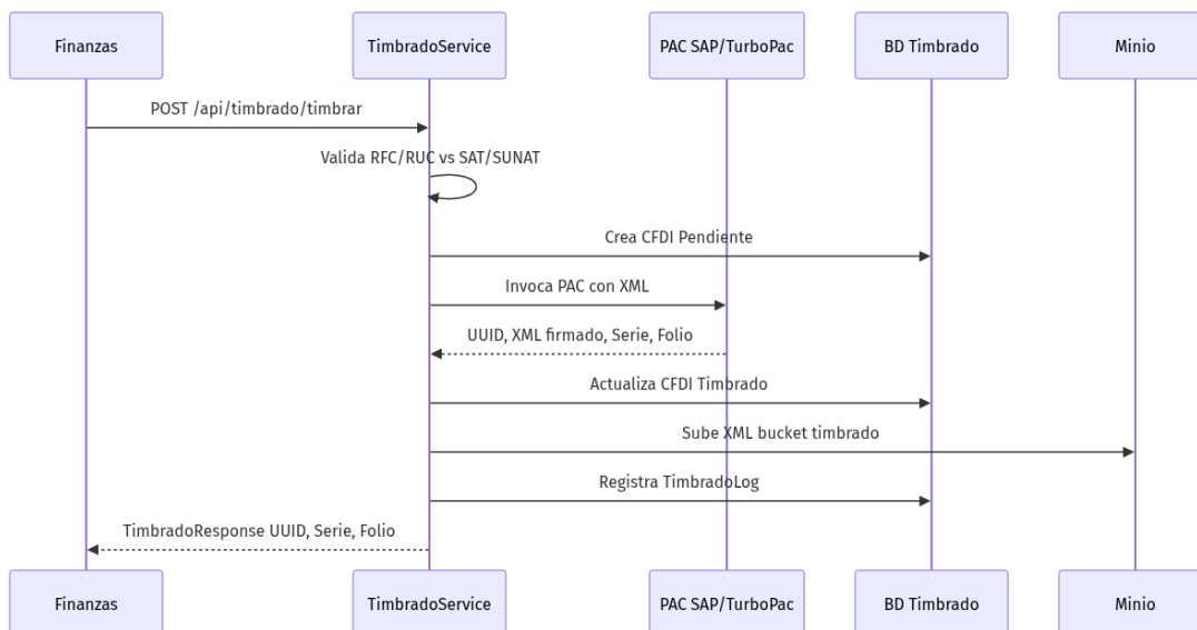
Diagrama 5 — Flujo de timbrado sincrónico (Sequence)
