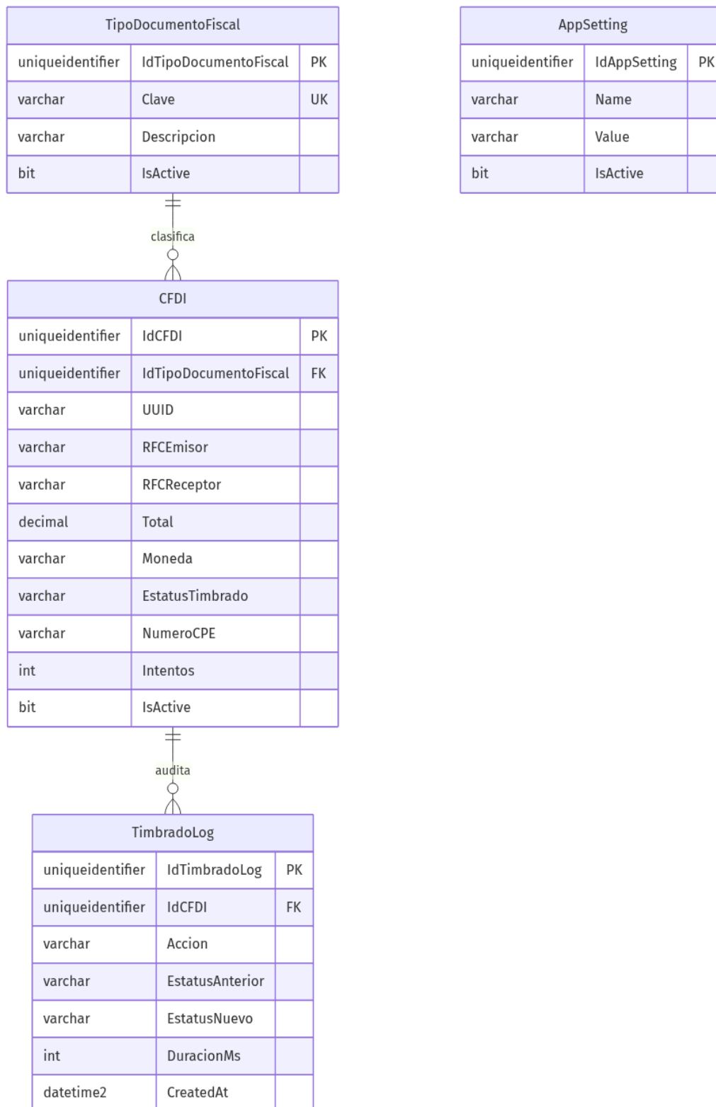
Diagrama 4 — Modelo de datos ProquifaDotNetTimbrado (ERD)
