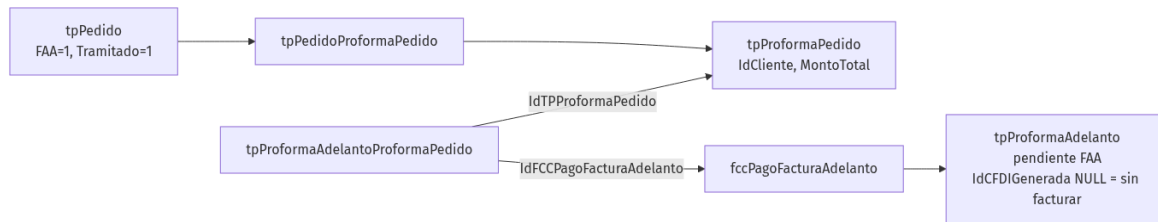
Diagrama 2 — Cadena de datos FAA en ProquifaDotNet (lectura)
