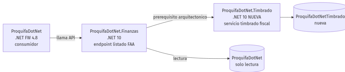
Diagrama 2 — Cadena de datos FAA en ProquifaDotNet (lectura)
